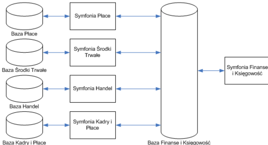
Model wymiany danych gdy programy Symfonii wykorzystują obiekt integracji.
